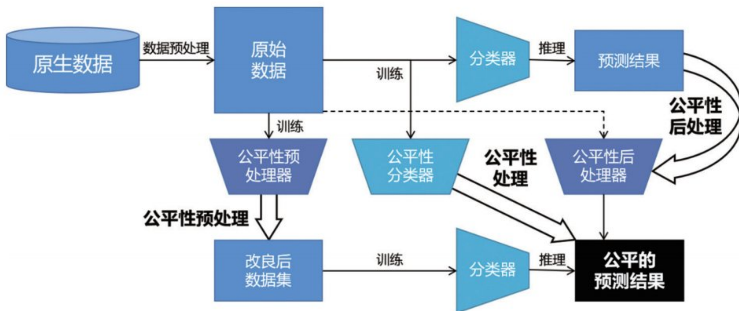
图4 公平机器学习流程
